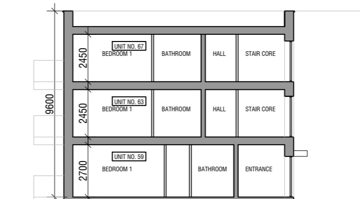
SECTION E2 SCALE 1:200
